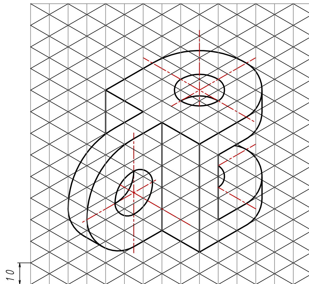
等角図
