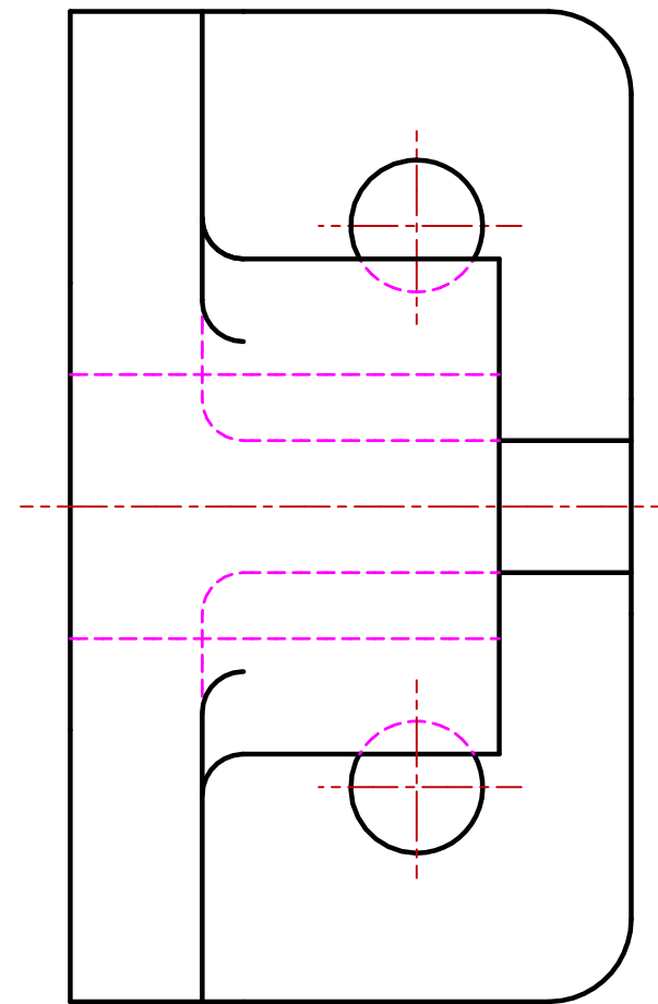
平面図（参考）
